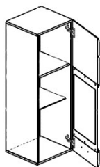
Шкаф настенный SFW1W P 38/110/35 шир./выс./гп.
