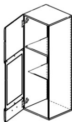
Шкаф настенный SFW1W L 38/110/35 шир./выс./гп.
